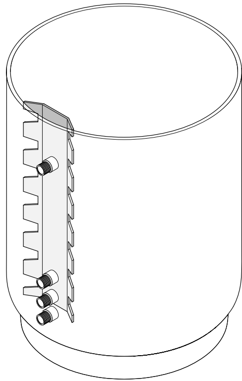
Abb. 3 Unterer Speicherbereich (geschnitten) mit innenliegendem Strömungsleitblech.
