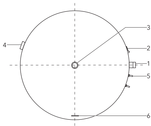
Abb. 2 RATIO Pufferspeicher - Draufsicht:
